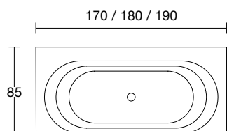
art. OASI33F - art. OASI34FC - art. OASI35FC
